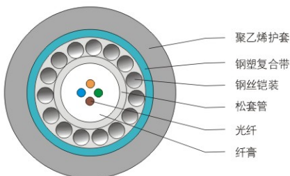
F-GYXTS型光缆典型截面图
