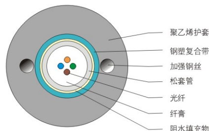
F-GYXTW型光缆典型截面图
