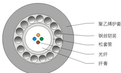
F-GYXTY 型光缆典型截面图
